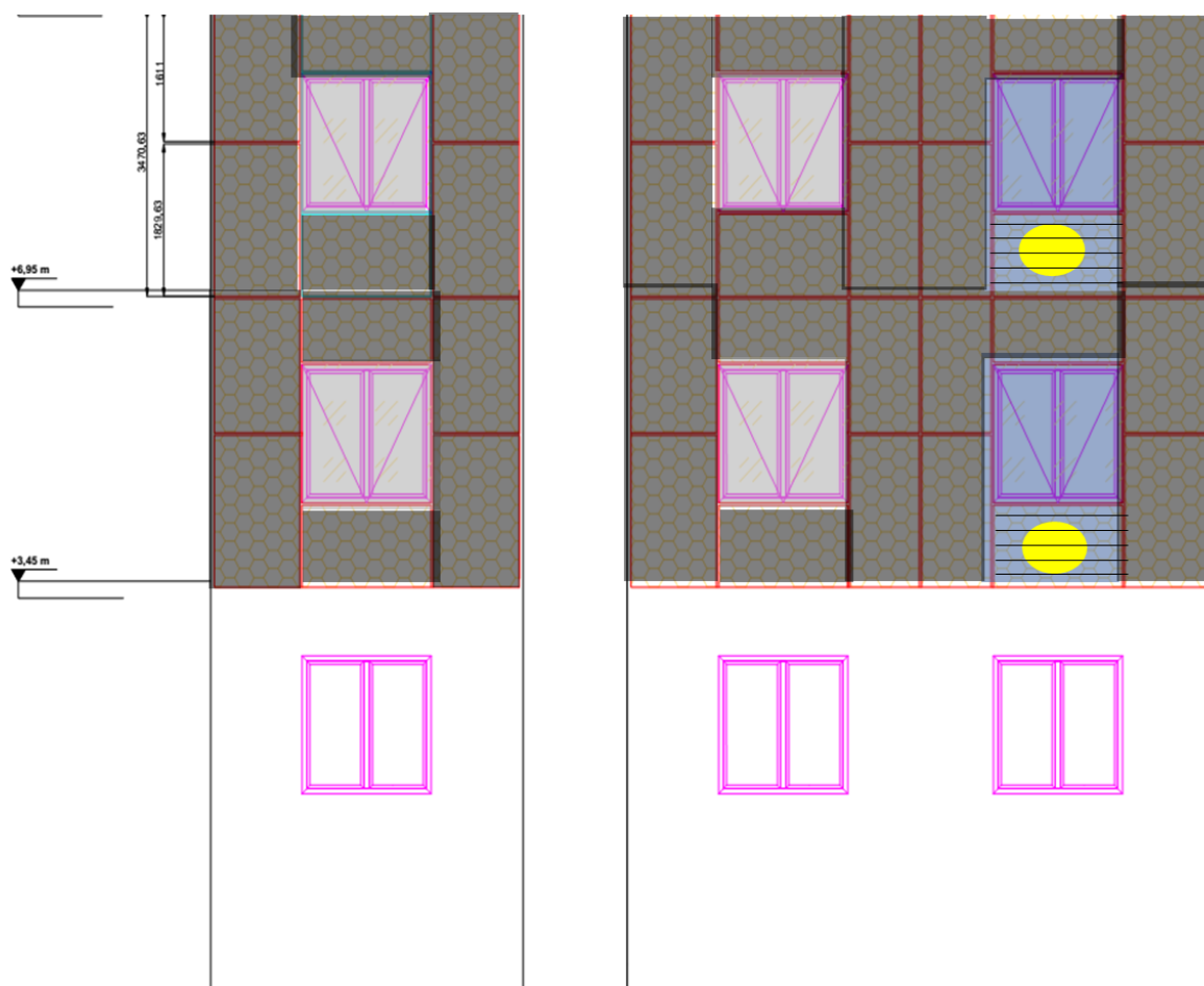
Εικόνα 8: Διάγραμμα της πρόσοψης με σημειωμένη τη θέση των συστημάτων ανάκτησης θερμότητας
