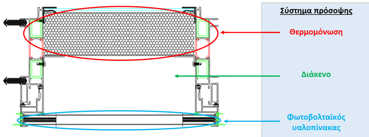
Εικόνα 5: Κάτοψη του συστήματος πρόσοψης με τα επιμέρους στοιχεία (προφίλ αλουμινίου, θερμομόνωση, ΦΒ υαλοπίνακας)
