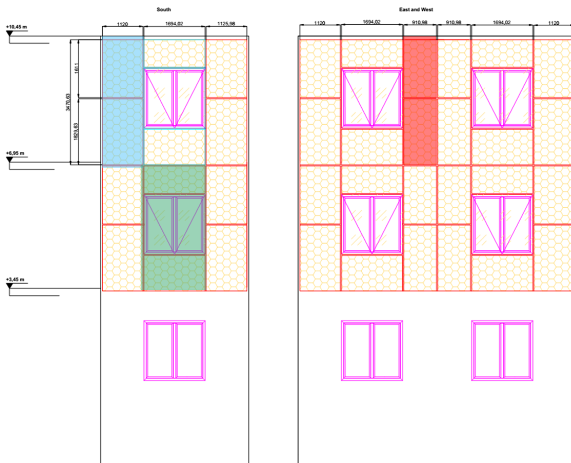
Εικόνα 6: Διάγραμμα κάλυψης της Νότιας (αριστερά) και ΝΑ/ΝΔ πλευράς (δεξιά) με τα πλαίσια των διαφόρων διαστάσεων
